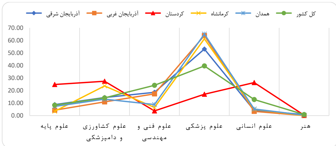
شکل ۳: تعداد پروژه‌های تحقیق و توسعه کارگاه‌های دارای فعالیت تحقیق و توسعه بر حسب گروه علمی
